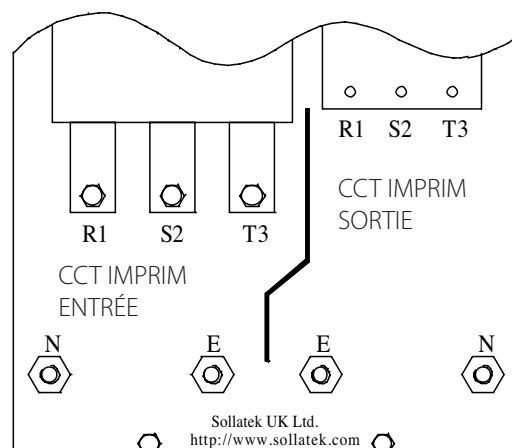
Schéma 2.6.1 Disposition typique des bornes
