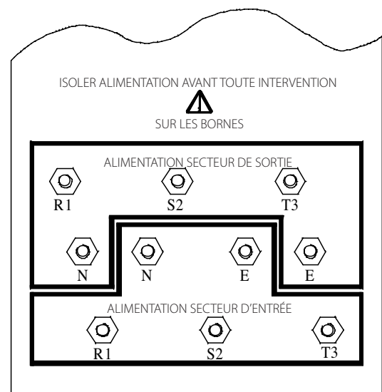
Schéma 2.6.1 Disposition des bornes
