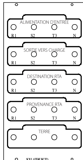
Figure 2 Repérage de la plaque à bornes du RTA
